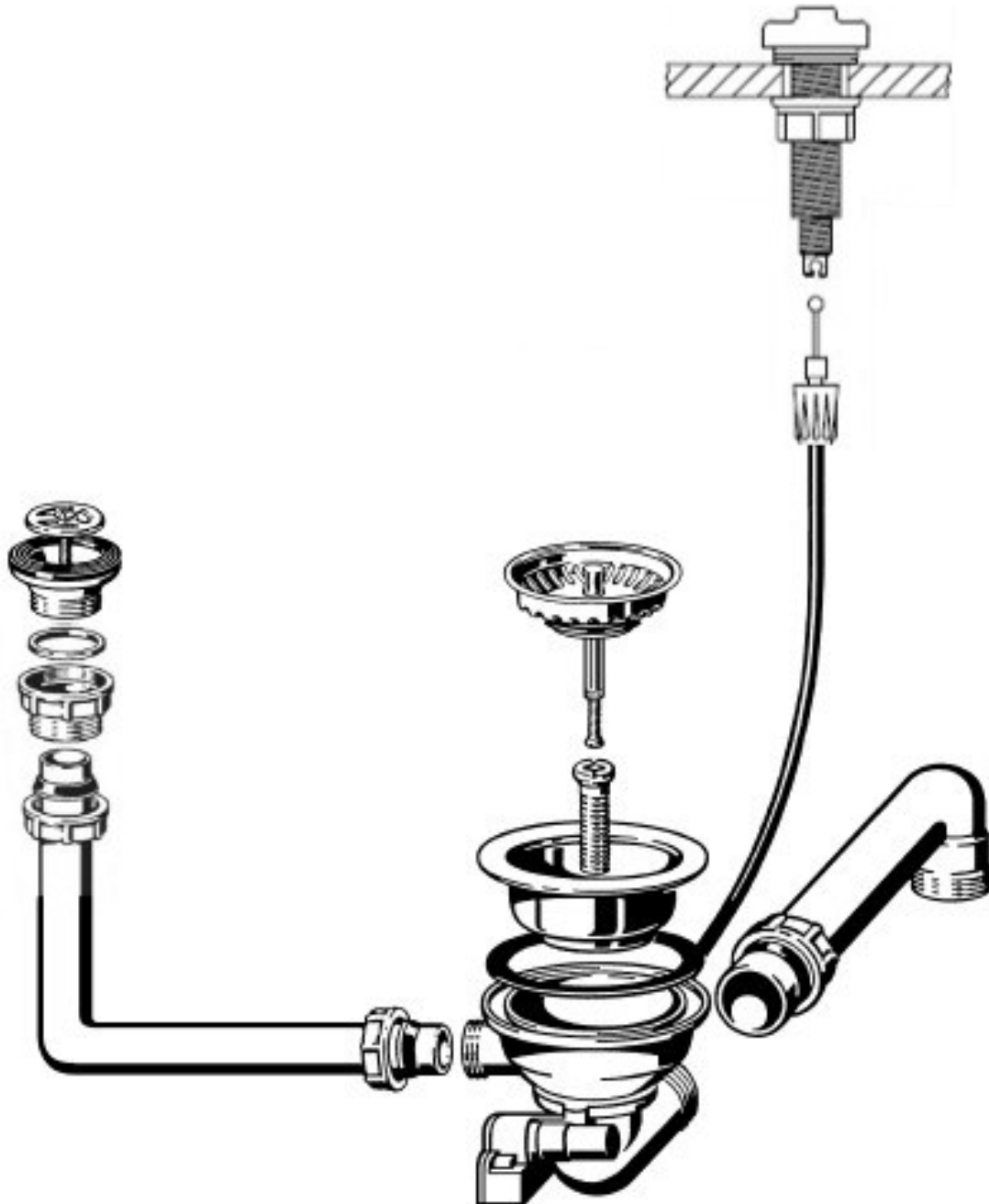
Ablaufgarnitur mit Excenterbetätigung 1 x 3 1/2"
