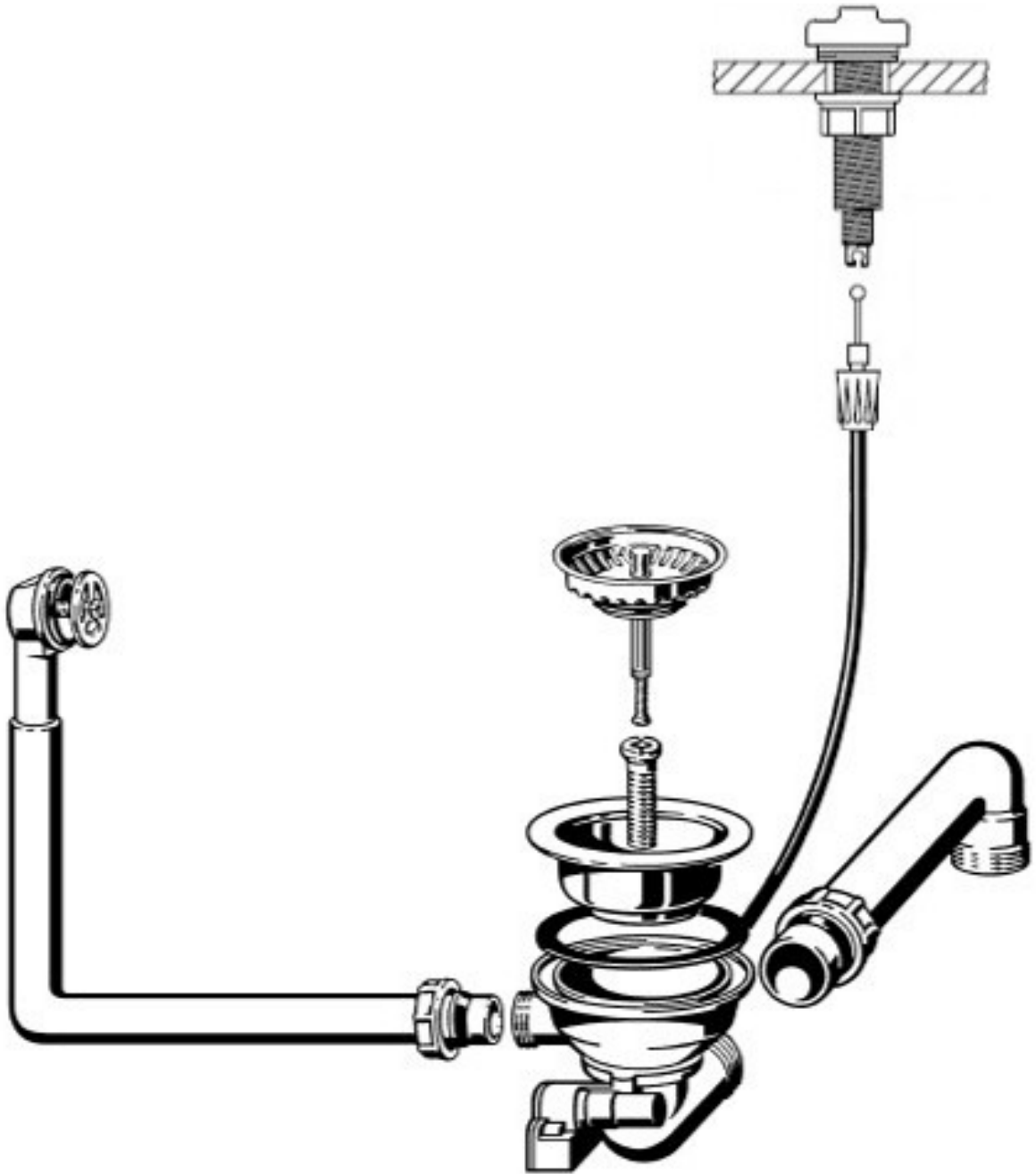
Ablaufgarnitur mit Excenterbetätigung 1 x 3 1/2"
